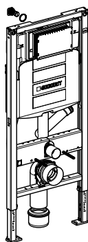
Duofix Wand-WC für Geruchsabsaugung, 112 cm, mit UP-Spülkasten UP320
