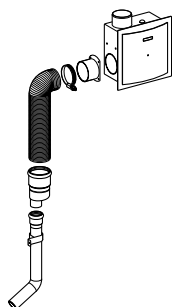
Geberit Aerotec90 Geruchsabsaugung zu UP320 mit Anschlussrohr und Einzellüfter
