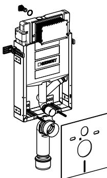
Kombifix Wand-WC für Geruchsabsaugung, mit UP-Spülkasten UP320
